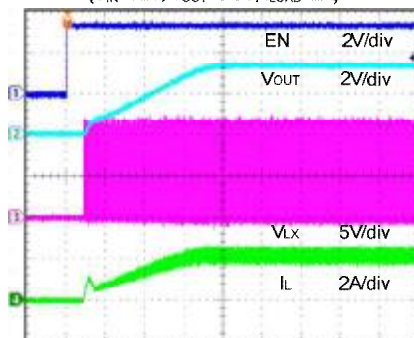
Startup
